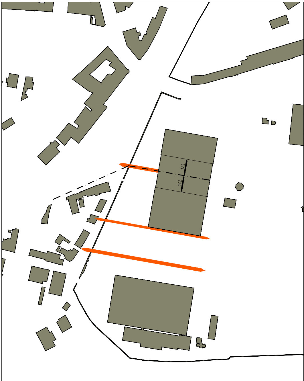
03. PŘÍČNÁ PRŮCHODNOST - propojení území s Pobřežní ulicí a vstupním předprostorem haly i obslužnými vstupy do jejího zázemí, průchody plotem v průhledu ulice u splavu, v pokračování jižní fasády haly a stromořadí u parkovací plochy
