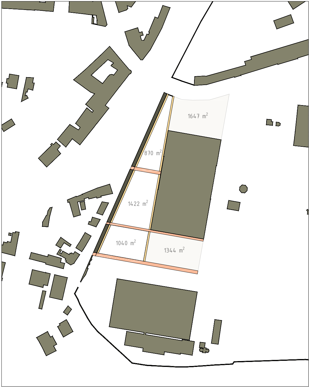
05. KOMUNIKAČNÍ SÍŤ - příčné stezky z hrubých dubových prken a podélné stezky z košťatovaného betonu dělí území na podobně velké části, v místě plotu do Pobřežní ulice vzniká nový úzký dům, který do sebe pojímá veškeré potřebné zázemí
