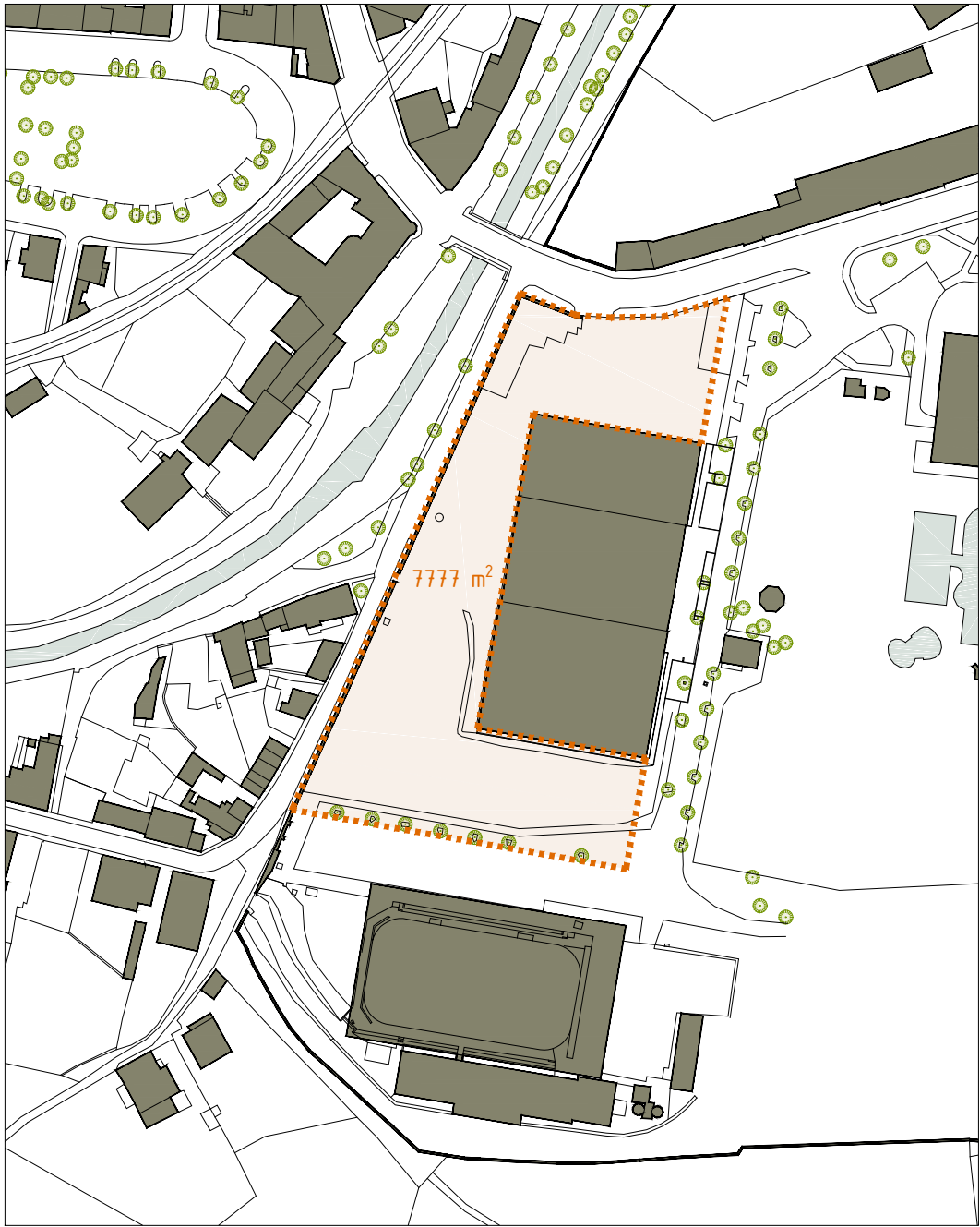
01. ŘEŠENÉ ÚZEMÍ - vymezení třemi bočními fasádami sportovní haly, jejím vstupním předprostorem, chodníkem do Čáslavské ulice, zděným plotem do ulice Pobřežní a stromořadím javorů směrem k asfaltovému parkovišti u zimního stadionu
